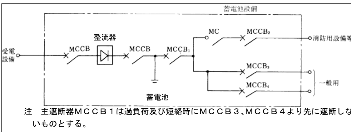
《主遮断器の二次側より分岐する例》
